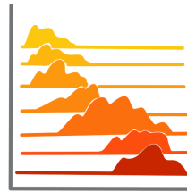
RIDGEPLOT
