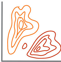
KDE PLOT
